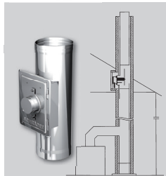
Montage des Feinstaubabscheiders im Gebäude
